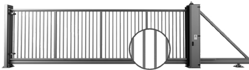
Das Schiebetor mit einer Füllung in Form von geschlossenen Profilen von 25 x 25 [mm], die zu einer Konstruktion geschweißt werden – Ansicht von der Grundstückseite.
