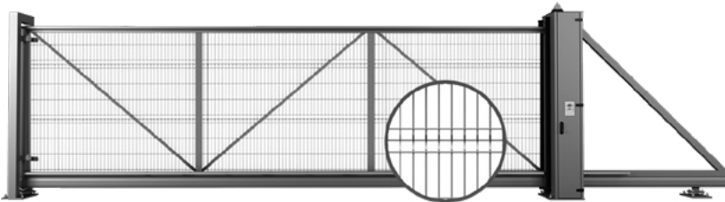
Schiebetor mit Füllung aus VEGA B Gittermatten, die an die Konstruktion angeschraubt sind – Ansicht vom Grundstück aus.
