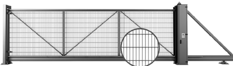
Schiebetor mit Füllung aus VEGA 2D Super Gittermatten, die an die Konstruktion angeschraubt sind – Ansicht vom Grundstück aus.
